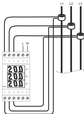
Версія з трансформатором струму
