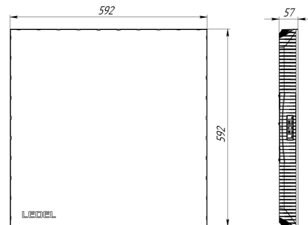
Рисунок 1 Светильник «L-office 32 Premium/Em»
