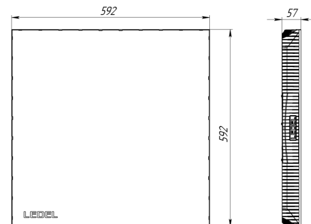
Рисунок 1 Светильник «L-office 55 Premium/Em»
