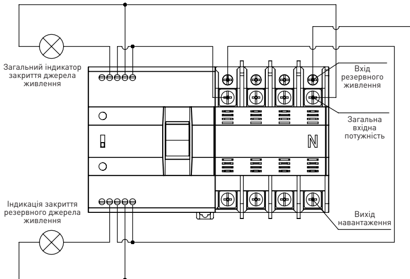
Рис. 6 Схема підключення для e.stand.ats.4.63
