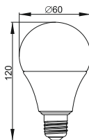
Рисунок 3 – Лампа LED-A60, 9 Вт, 11 Вт, цоколь E27
