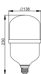
Рисунок 32 – Лампа LED-HP, 50 Вт, цоколь E27
