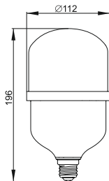
Рисунок 28 – Лампа LED– HP, 30 Вт, цоколь E27
