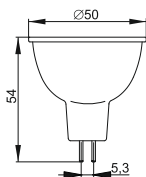
Рисунок 18 – Лампа LED–MR16, 9 Вт цоколь GU5.3
