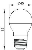
Рисунок 13 – Лампа LED–G45, 5 Вт цоколь E27
