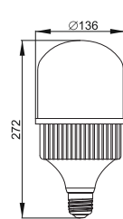
Рисунок 35 – Лампа LED-HP, 80 Вт, 100 Вт, цоколь E40
