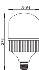
Рисунок 34 – Лампа LED-HP, 65 Вт, цоколь E40
