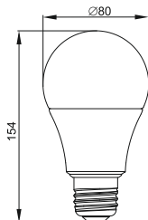
Рисунок 37 – Лампа LED- A80, 25 Вт цоколь E27
