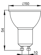
Рисунок 19 – Лампа LED–PAR16, 5 Вт цоколь GU10
