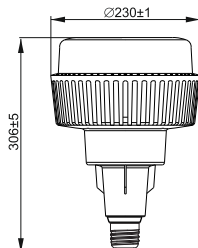
Рисунок 38 – Лампа LED- HP, 160 Вт, цоколь E40
