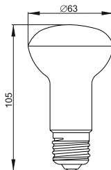
Рисунок 23 – Лампа LED–R63, 5 Вт, 8 Вт цоколь E27
