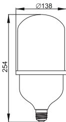
Рисунок 33 – Лампа LED-HP, 50 Вт, цоколь E40
