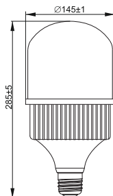
Рисунок 40 Лампа LED- HP, 120 Вт, цоколь E40
