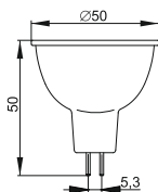
Рисунок 17 – Лампа LED–MR16, 7 Вт цоколь GU5.3
