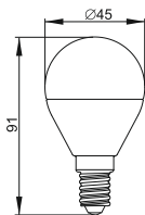
Рисунок 14 – Лампа LED–G45, 7 Вт, 9 Вт, цоколь E14
