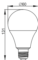
Рисунок 2 – Лампа LED-A60, 13 Вт, 15 Вт, 20 Вт цоколь E27
