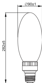
Рисунок 39 – Лампа LED- HP, 35 Вт, 60 Вт, цоколь E40
