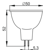
Рисунок 16 – Лампа LED–MR16, 3 Вт, 5 Вт цоколь GU5.3
