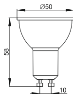
Рисунок 20 – Лампа LED–PAR16, 7 Вт цоколь GU10
