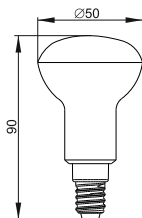
Рисунок 22 – Лампа LED–R50, 5 Вт цоколь E14
