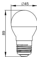
Рисунок 15 – Лампа LED–G45, 7 Вт, 9 Вт, цоколь E27
