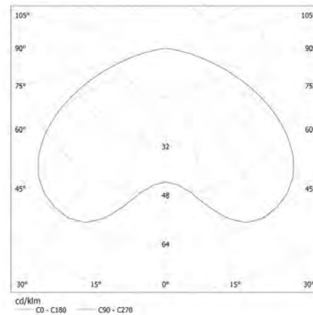
KANLUX S.A. (kat 7195) XARD DL-40 / Krzywa rozsytu światła (biegunowo) Оправа: KANLUX S.A. (kat 7195) XARD DL-40 Лампы: 1 x TC-QSE 16W/827
