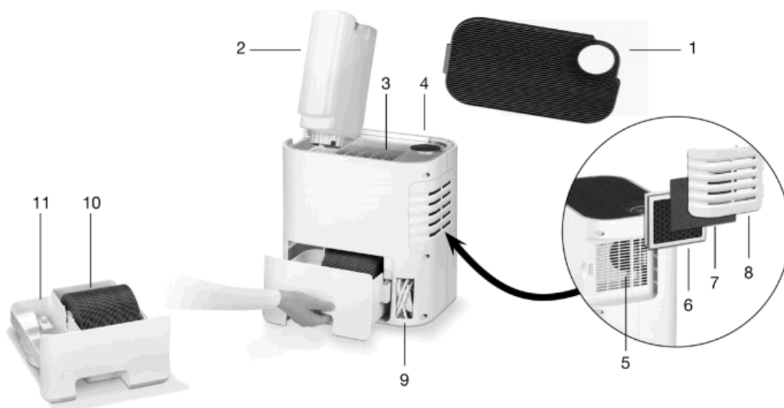
Малюнок 1 – Конструкція кліматичного комплексу МР-50
