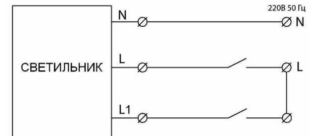
Рисунок 3 Схема подключения светильника
