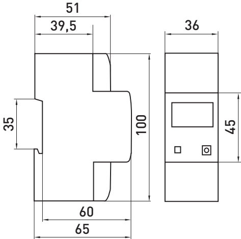
Рис. 1 Габаритні розміри
