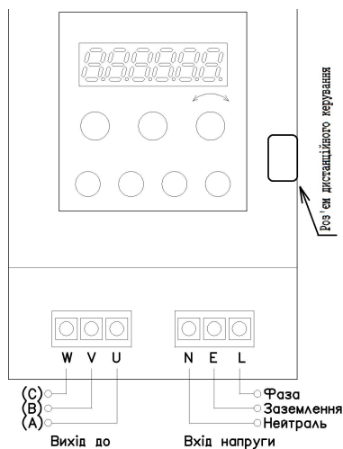
Мал. 1. Схема електричних з'єднань.
