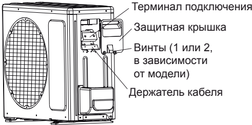
Терминал подключения проводов
