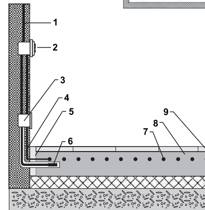
Конструкція підлоги з підігрівом
