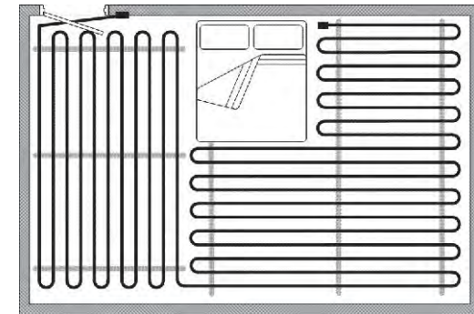
Конструкція підлоги з підігрівом
