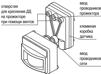
Рисунок 16. Конструкция датчика движения ДД017
