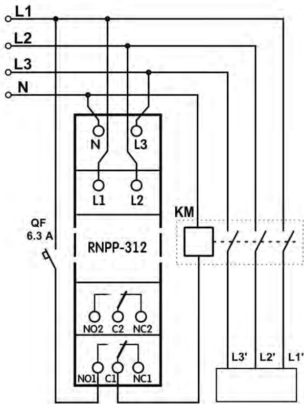
Рисунок 2 – Схема подключения RNPP-312
