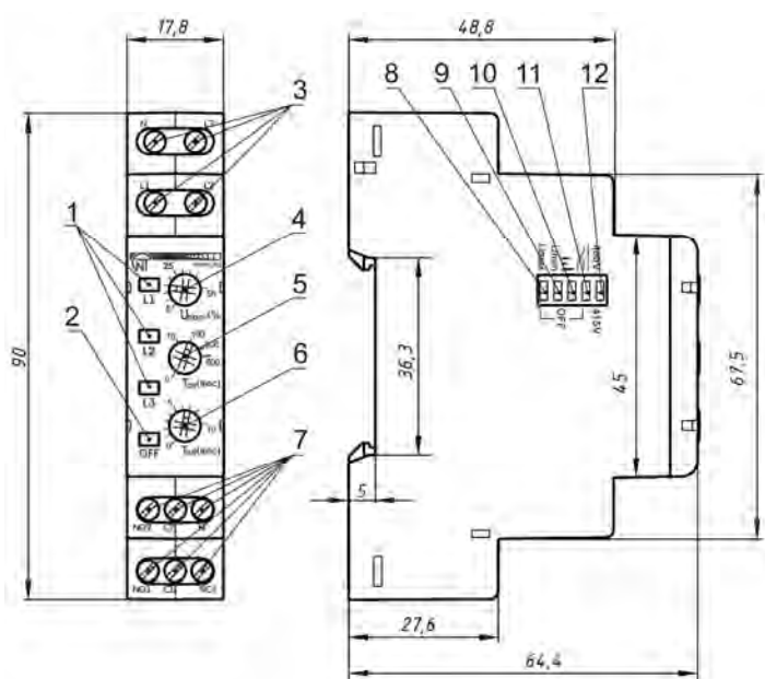
Рисунок 1 – Органы управления, габаритные и установочные размеры RNPP-312
