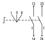
Переключатель LA167-BDF33
