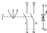
Переключатель D8-20XD3
