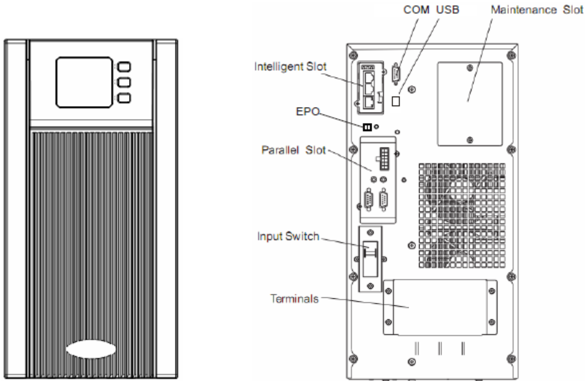
Рис.1 6 кВА (Н) Вид передней панели Рис. 2 6 кВА (Н) Вид задней панели
