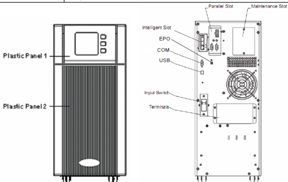
Рис.7 10 кВА (С) Вид передней панели Рис.8 10 кВА (С) Вид задней панели
