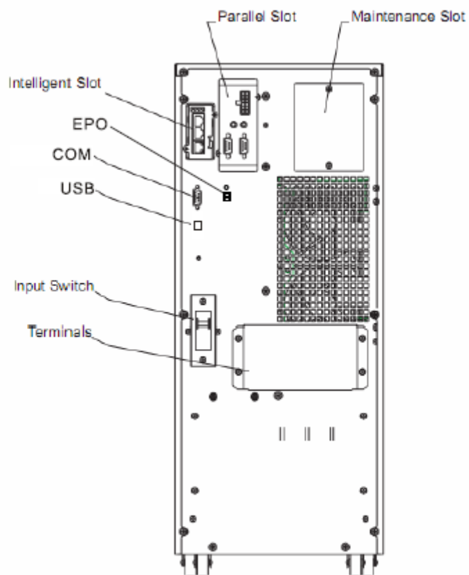
Рис.4 6 kVA (S) Вид задней
