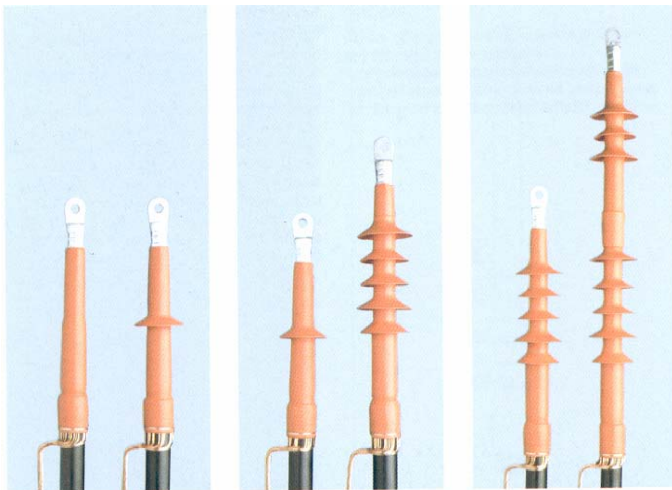
Внутренняя и наружная установка на 35 кВ
