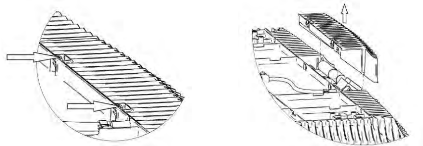
Рисунок 2 Снятие декоративной крышки драйверного отсека
