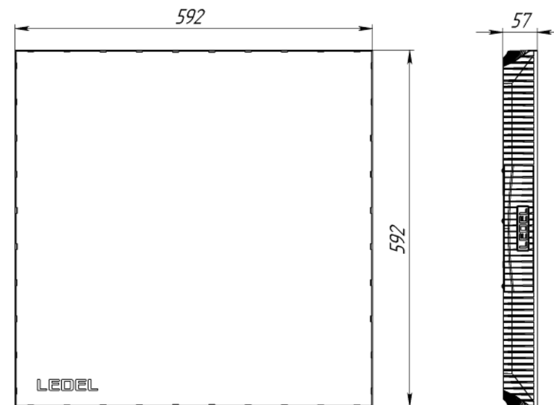
Рисунок 1 Светильник «L-office 32 Standart», «L-office 55 Standart»
