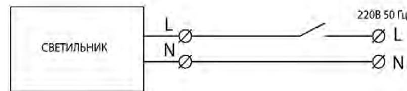
Рисунок 3 Схема подключения светильника
