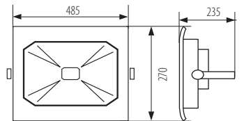
ANTRA LED150W
