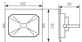
ANTRA LED100W
