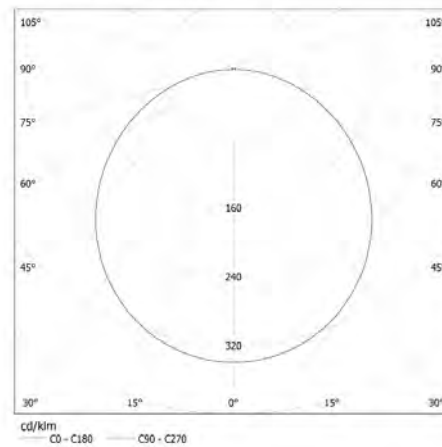
KANLUX S.A. (kat 25790) TOWE LED 36W-NW / Krzywa rozsytu światła (biegunowo)
