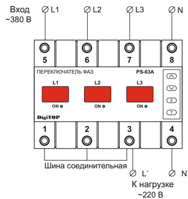
Схема подключения
