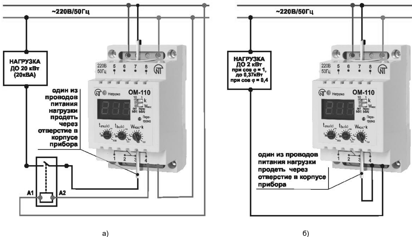
Рисунок 2 - Схема подключения ОМ-110
