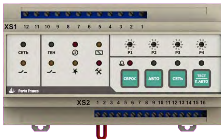
Рис. 5.2. Конфигурация контроллера
