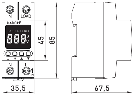
Рис. 1 Габаритні розміри
