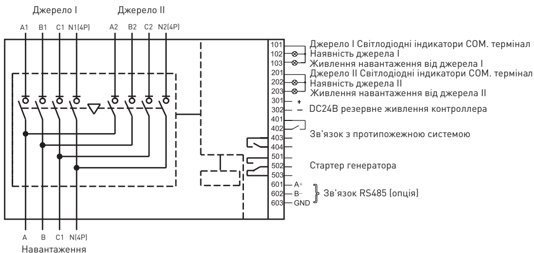
Рис. 5 Схема підключення АВР
