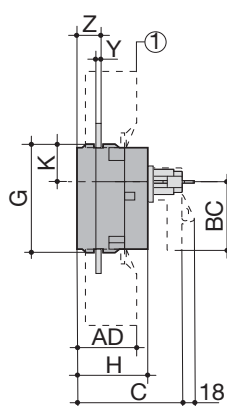
Выносное фронтальное управление Вид сбоку
