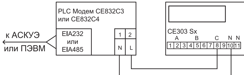
Рисунок 3.9 – Схема подключения счетчика
