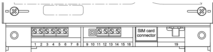
в) обозначение контактов счетчика CE303 S3x для исполнений со встроенным GSM-модулем контакты 1,2 – подключение импульсных выходов TM1 (P); контакты 3,4 – подключение импульсных выходов TM2 (Q); контакт 5 – подключение (+) РИП (9-24 В – для исполнений счетчика со встроенным GSM-модулем,
