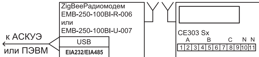
Рисунок 3.8 – Схема подключения счетчика
