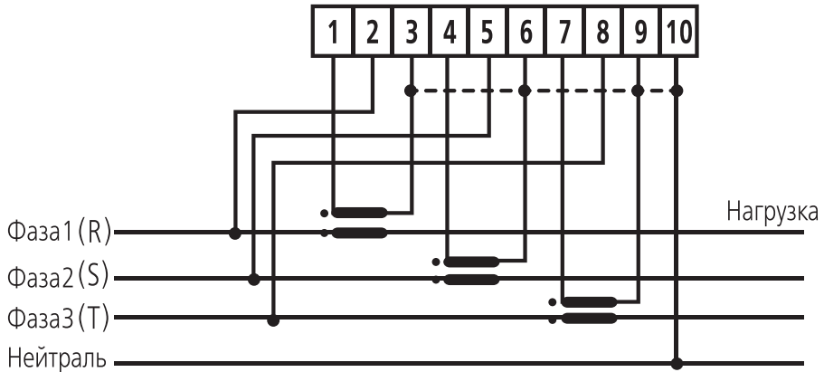
Схема включения счетчика СЕ303 230В 5(10)А Подключение через три трансформатора тока (трехфазная четырехпроводная сеть)
