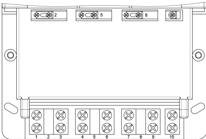
Рисунок 3.1 – Обозначение контактов счетчика исполнения СЕ303 SX
