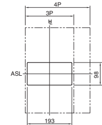
Вырезы в панели (вид спереди)
