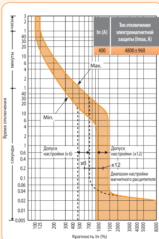
EB2 400 SF Характеристика t-I
