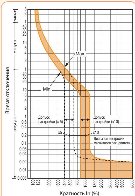
EB2 800/LF 800A Характеристика t-I
