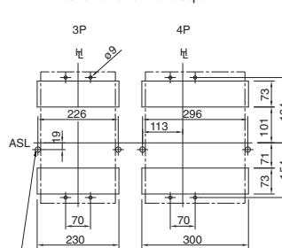
Разметка монтажных отверстий
