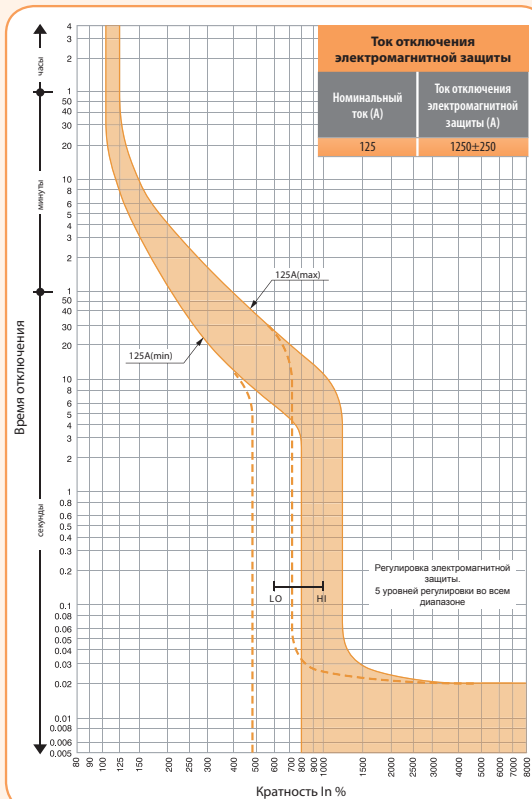
EB2 125 (125A) Характеристика t-I
