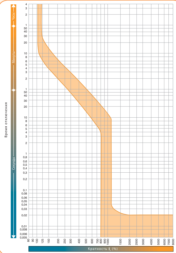
EB2R 250 (250A) Характеристика t-I
