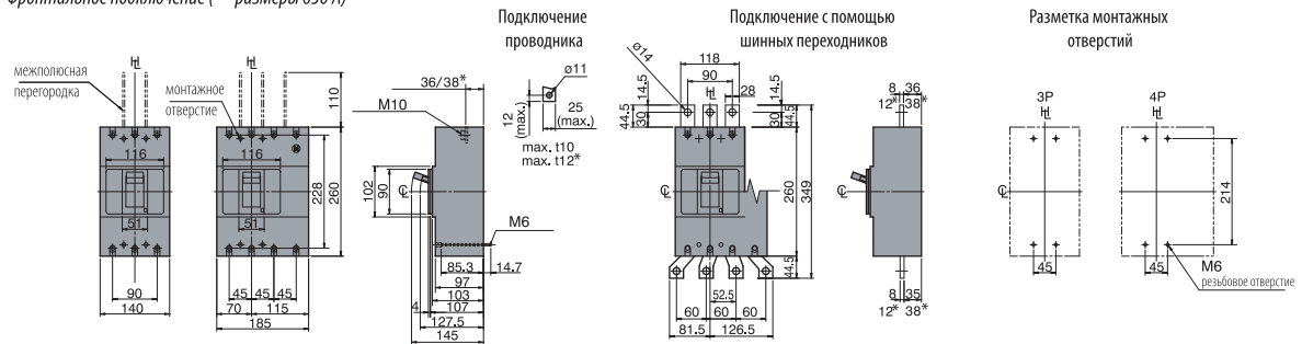
Фронтальное подключение (* - размеры 630 А)
