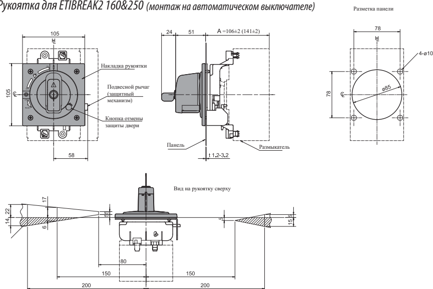
Рукоятка для ETIBREAK2 160&250 (монтаж на автоматическом выключателе)
