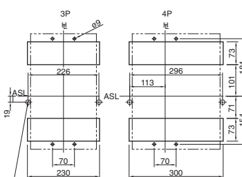
Разметка монтажных отверстий
