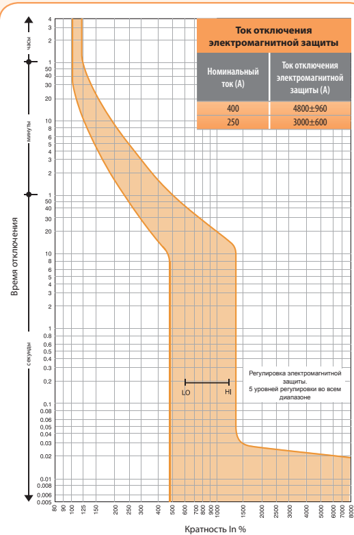
EB2 400 A Характеристика t-I
