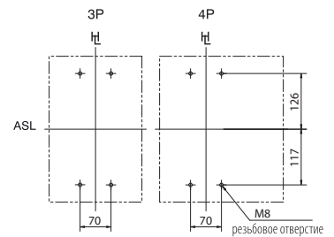
Разметка монтажных отверстий
