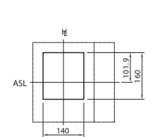
Вырезы в панели (вид спереди)
