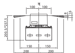
Положение петель (заштрихованная область) вид снизу
