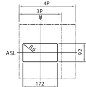
Вырезы в панели (вид спереди)
