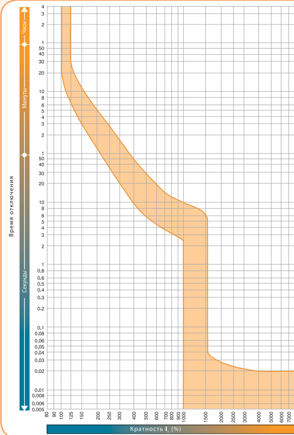
EB2R 250 (160A) Характеристика t-I
