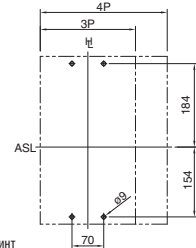
Разметка монтажных отверстий
