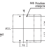
Разметка монтажных отверстий
