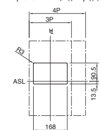
Вырезы в панели (вид спереди)
