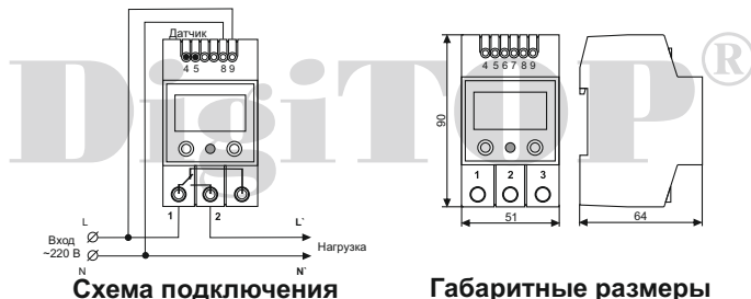
Схема подключения
