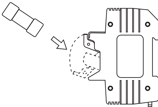
Рис. 2 Встановлення плавких вставок у пристрій
